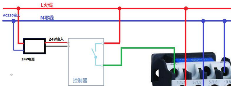
AC220V接线示意图 L代表火线 N代表零线
